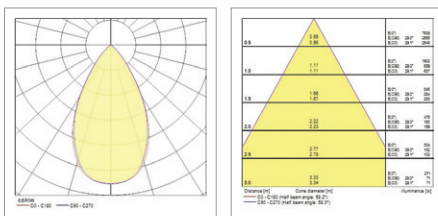
Pixo Zoom Multipower 25W 2700K 60°
