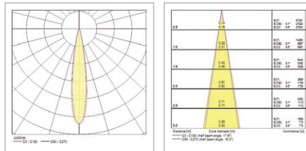
Pixo Zoom Multipower 25W 3000K 17°
