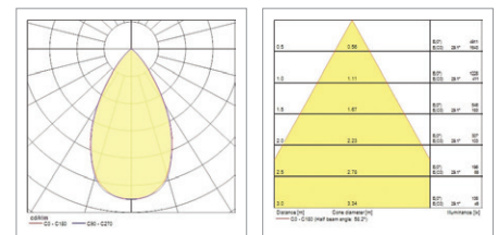
Pixo Zoom Multipower 12W 4000K 60°
