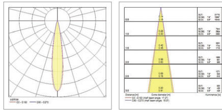
Pixo Zoom Multipower 12W 3000K 17°
