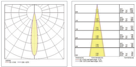
Pixo Zoom Multipower 12W 2700K 17°
