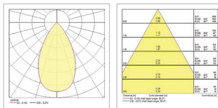
Pixo Zoom Multipower 12W 3000K 60°
