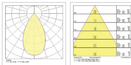
Pixo Zoom Multipower 25W 3000K 60°
