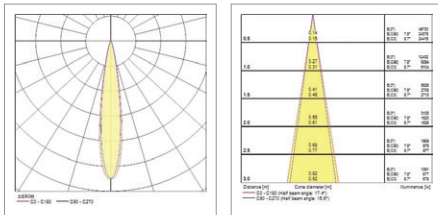
Pixo Zoom Multipower 25W 2700K 17°
