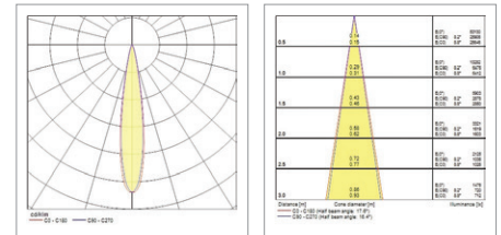
Pixo Zoom Multipower 25W 4000K 17°
