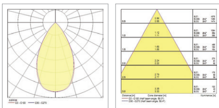
Pixo Zoom Multipower 12W 2700K 60°
