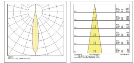
Pixo Zoom Multipower 12W 4000K 17°
