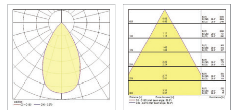
Pixo Zoom Multipower 25W 4000K 60°
